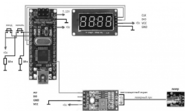
Рис. 1. Схема Arduino
